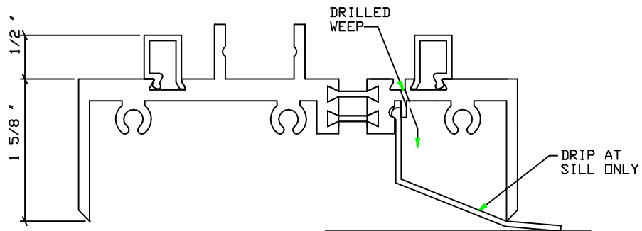
PERIMETER JAMB
